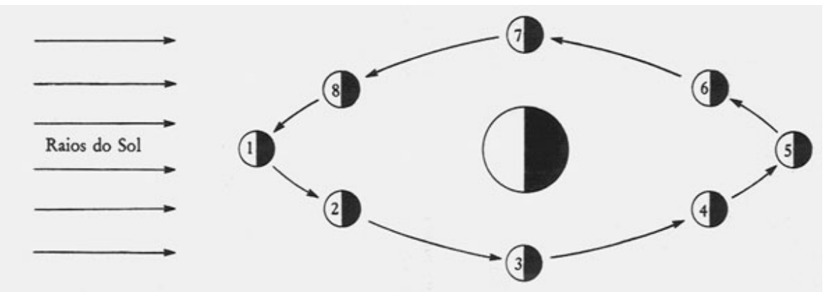
Fig. 1.3 ÓRBITA LUNAR
