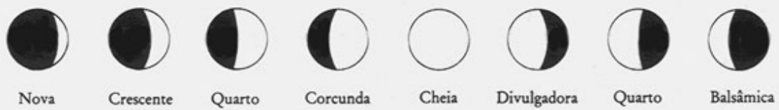
Fig. 1.4 FASES DA LUA
