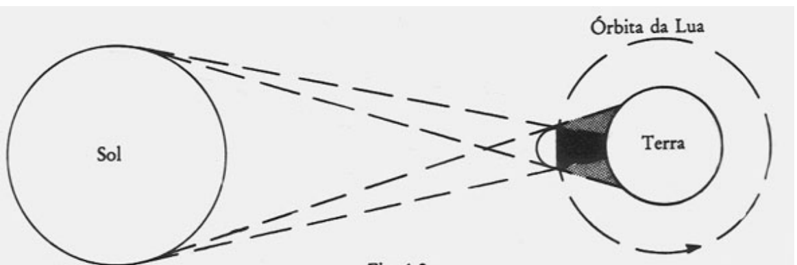
Fig. 1.2 ECLIPSE DO SOL
