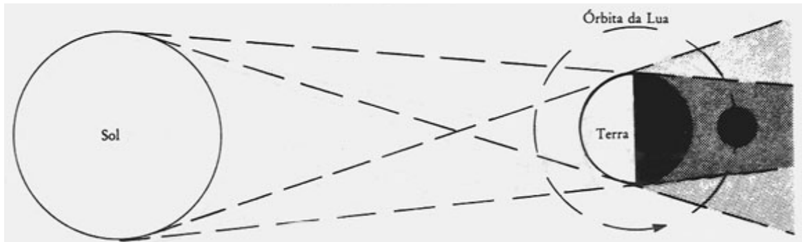
Fig. 1.1 ECLIPSE DA LUA
